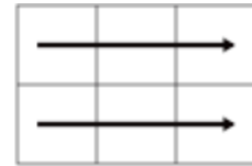
dot(A,B,2)
