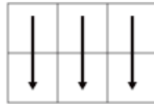
dot(A,B,1)
